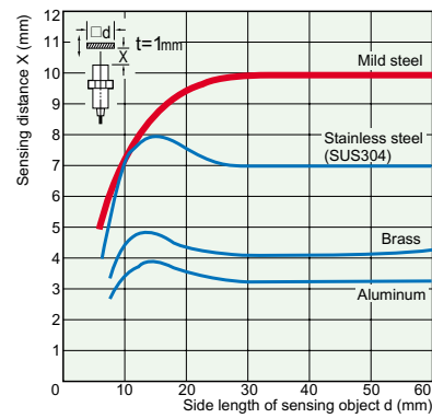
E2F-X10□□
