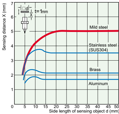
E2F-X5□□
