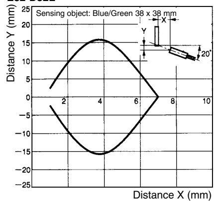
E32-D32L
