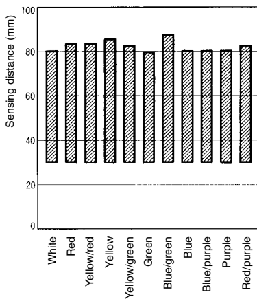
E3MC-(M)A□□
